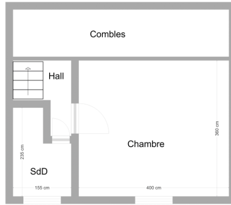
ETAGE 2
