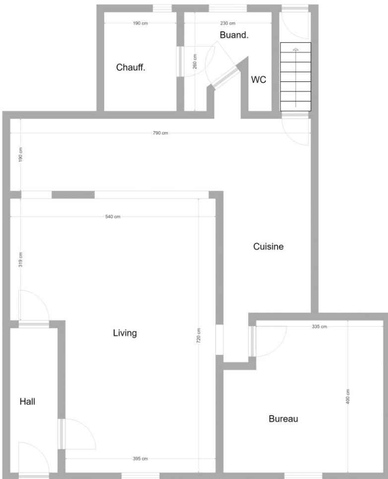
REZ-DE-CHAUSSEE
